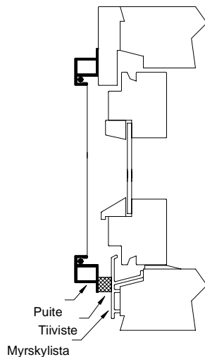
Pystyleikkaus
