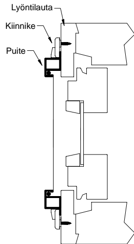
Vaakaleikkaus
